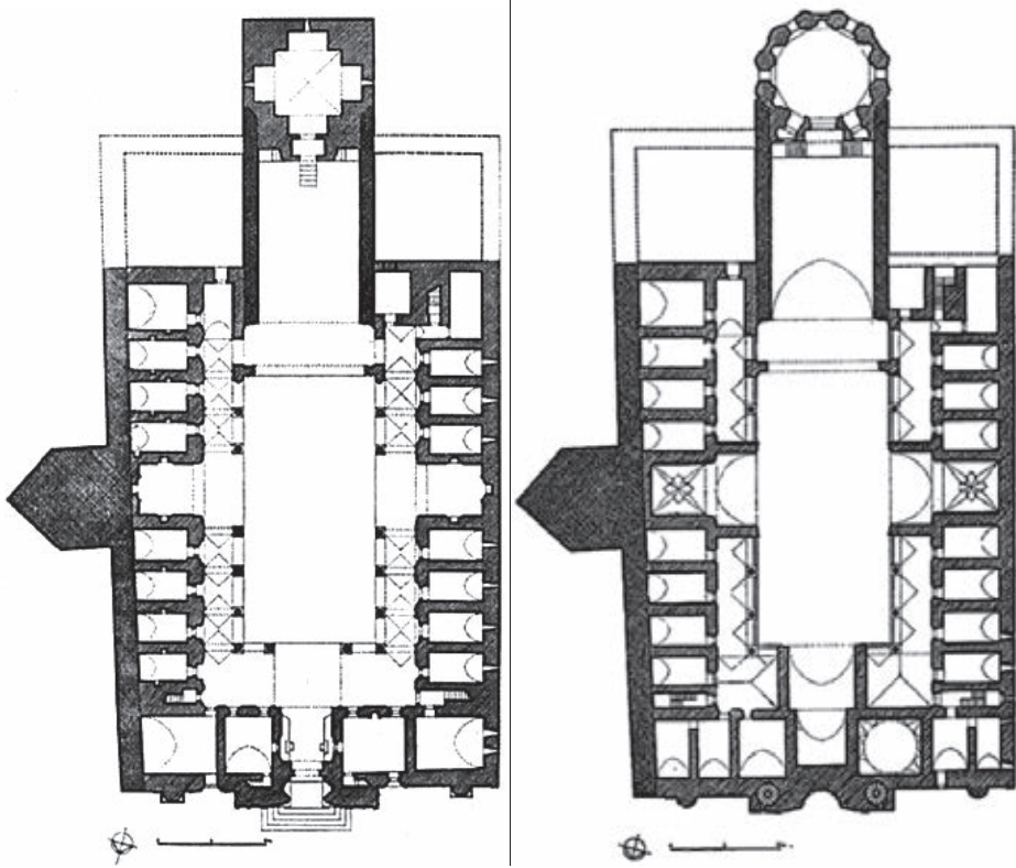
Leoha 2. Erzurum Çifte/Hatuniye Medresesi, alt ve üst kat planları 24
